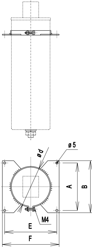
Clamp type C... / Держатель типа С...
