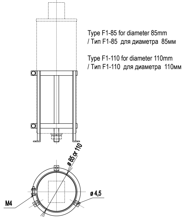
Clamp type F... / Держатель типа F...
