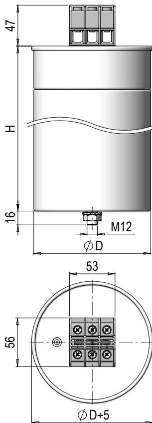
Drawing No./Габаритный чертёж 3b
