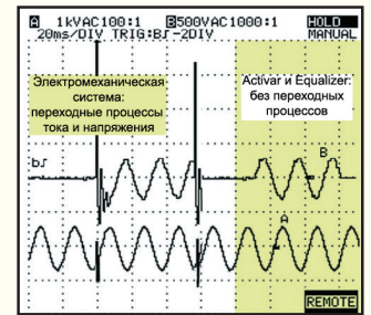
Электромеханическая коммутация в сравнении с коммутацией без переходных процессов
