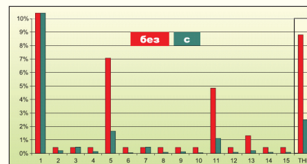
Пример фильтрации гармоник напряжения
