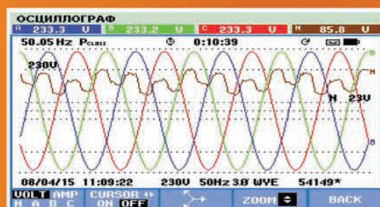
Выходное напряжение
